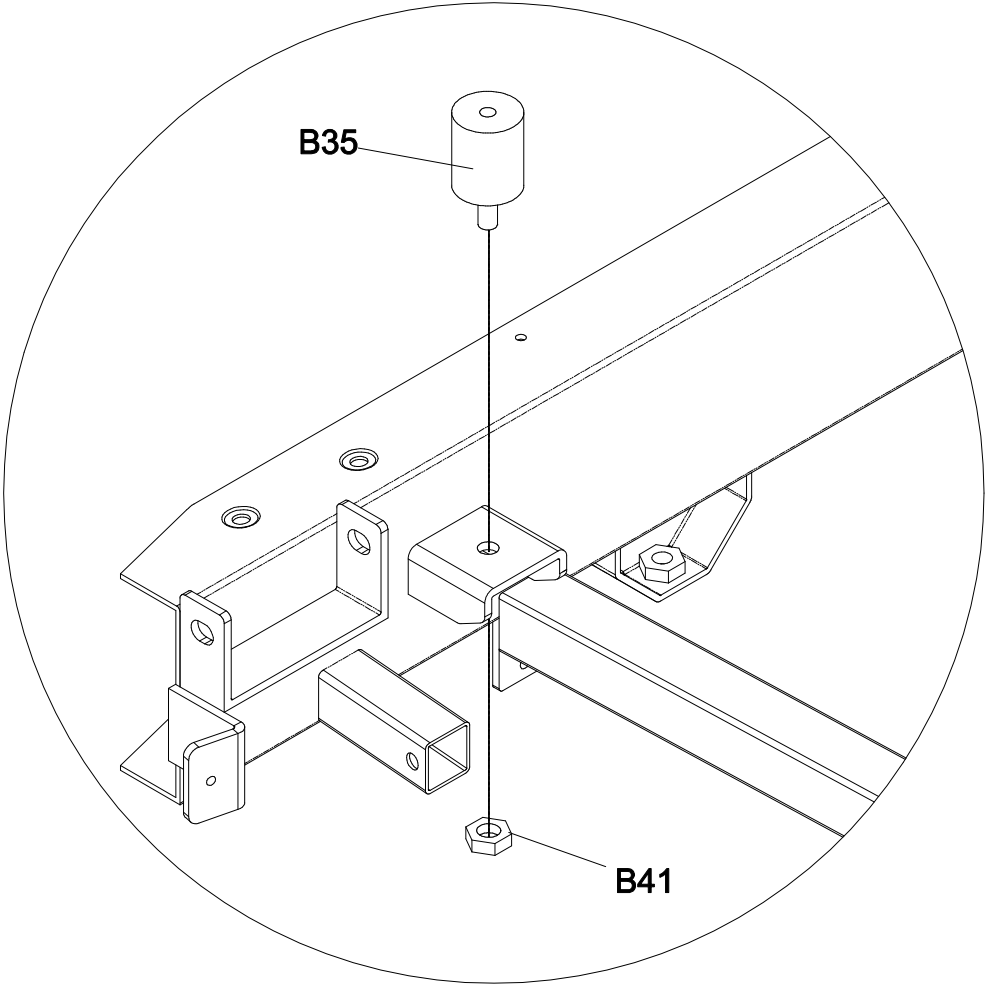
A詳圖(1:5)
